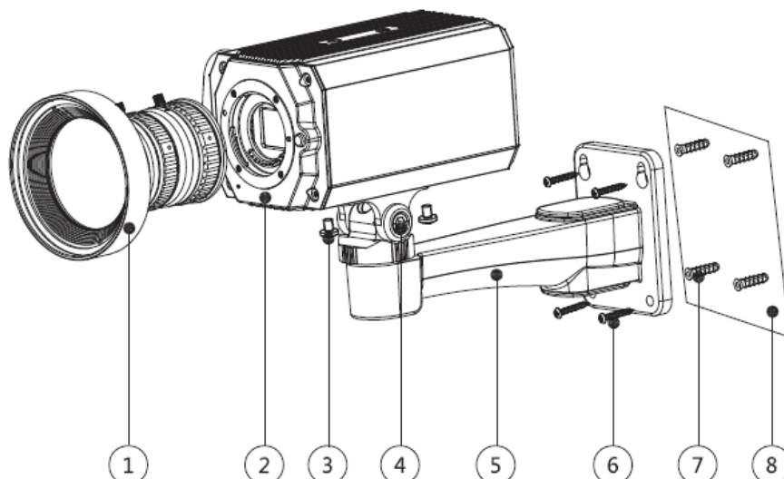
Figura 8-6 Componentes del dispositivo
