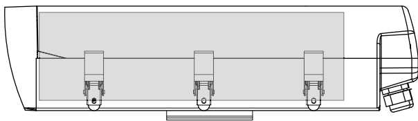
Dimensiones en mm para las carcasas de interior UHI-OG(S)-0
