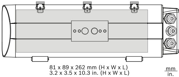
Espacio interior máximo disponible en mm (según el tamaño de lente/cámara)
