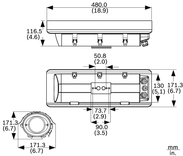
Dimensiones en mm para las carcasas de interior UHI-OG(S)-0
